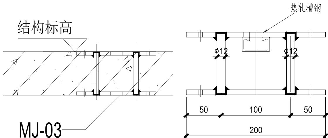
本工程18层室内埋板节点图与加工图
