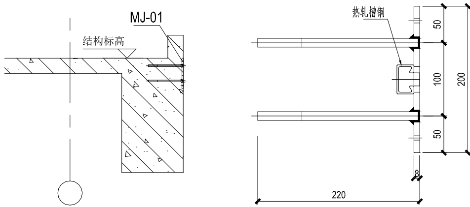
本工程“侧埋”埋板节点图与加工图
