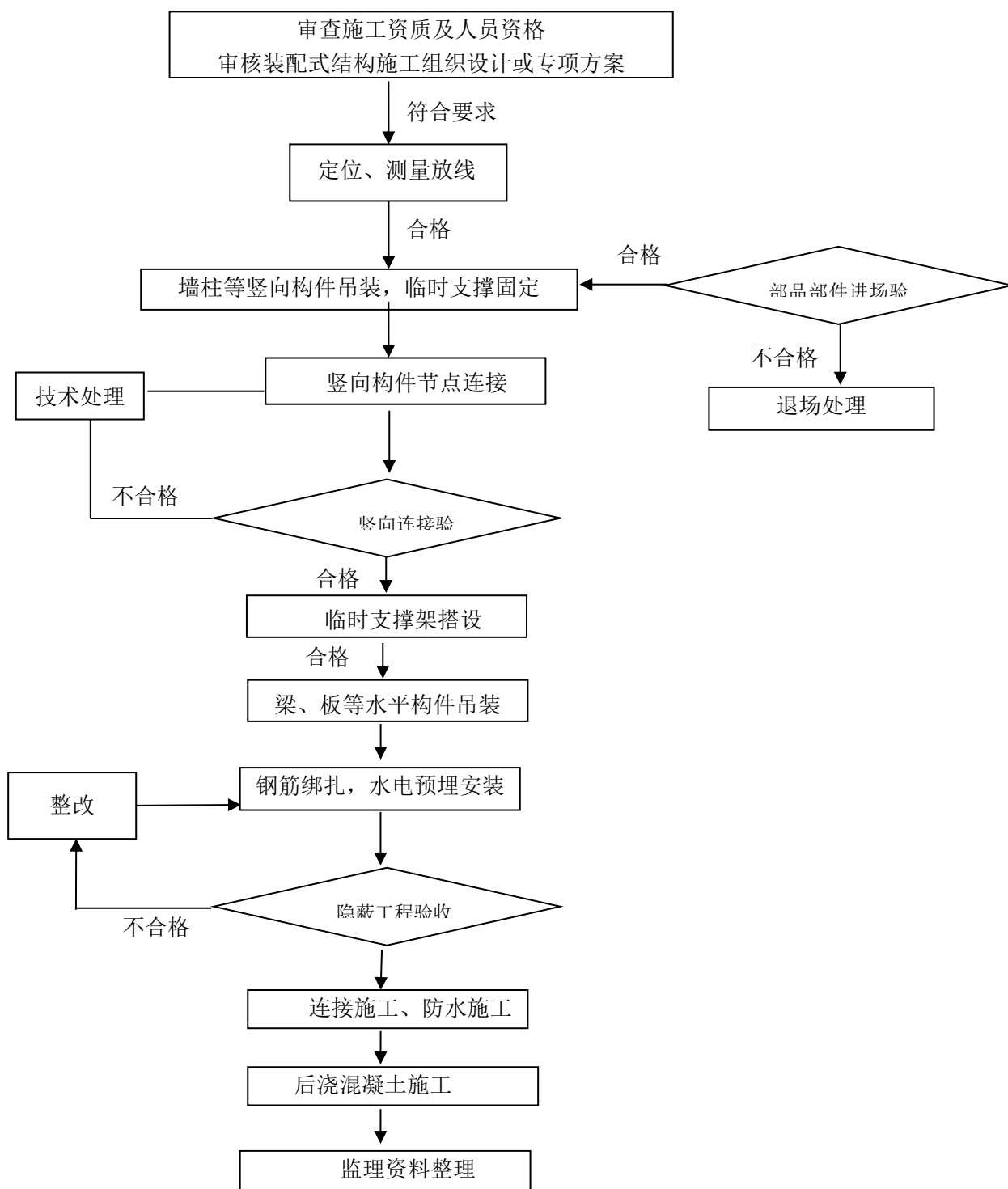
装配式混凝土结构施工监理程序框图
